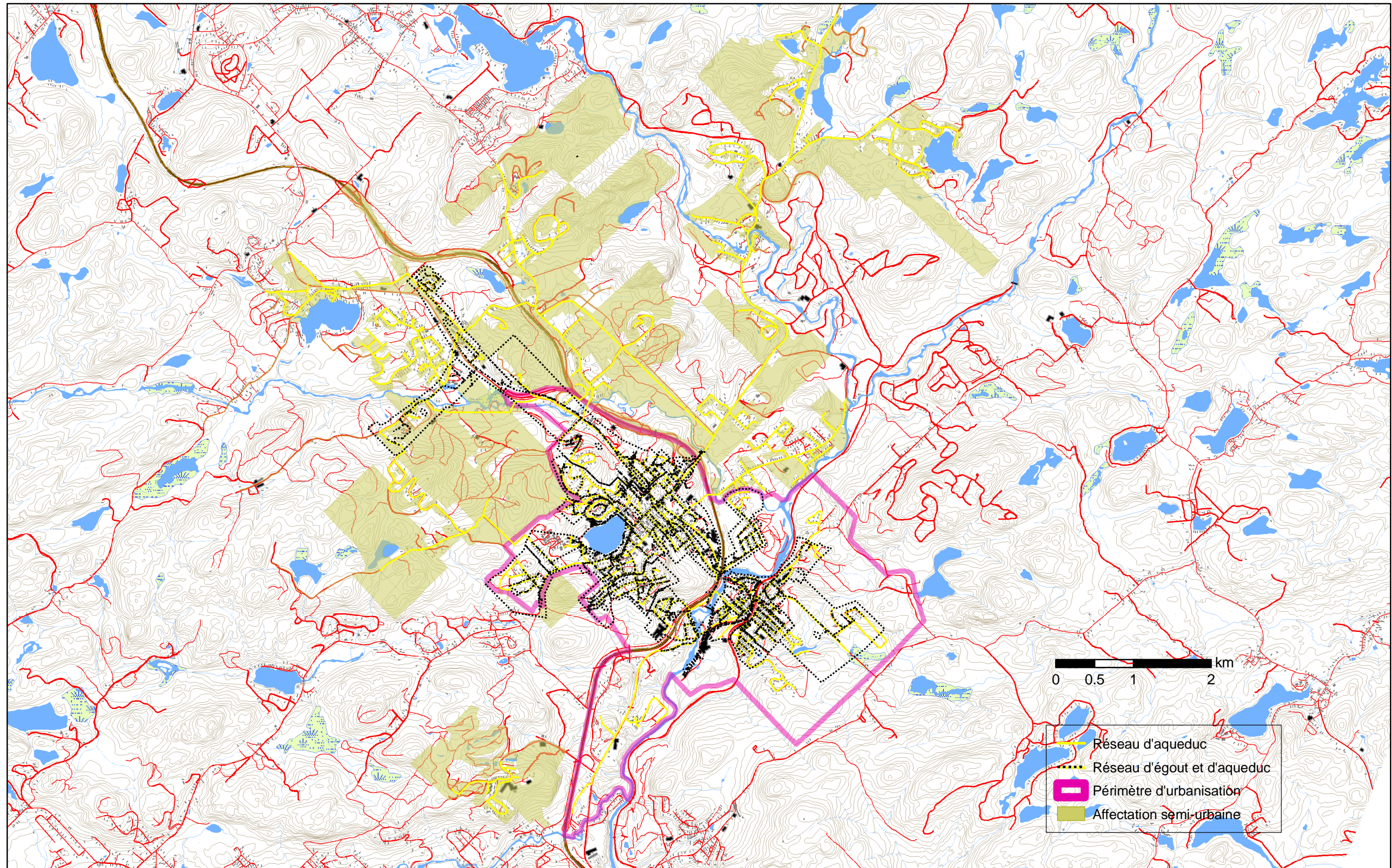
Carte 10 - Réseau d'aqueduc et d'égout Sainte-Adèle
